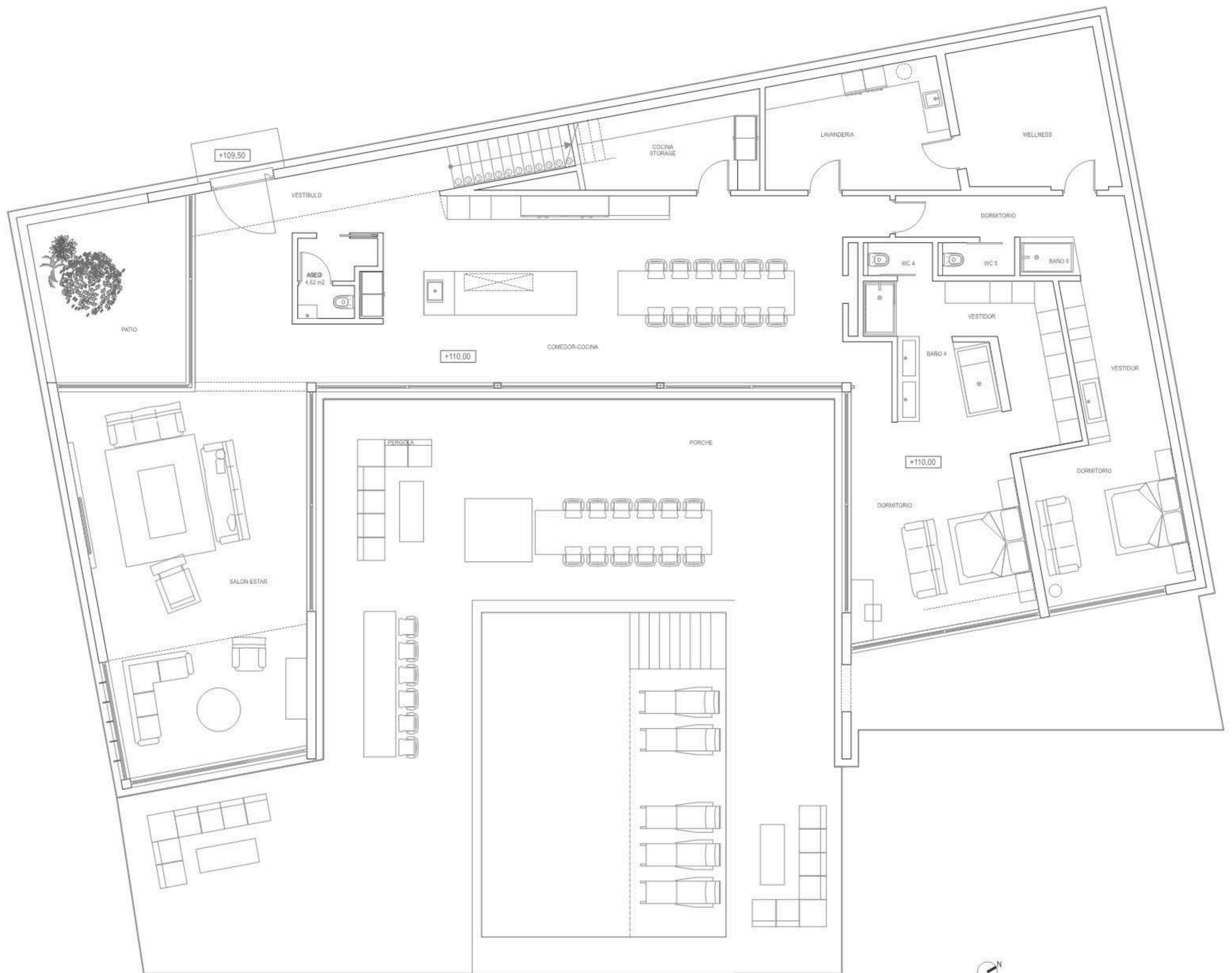
PLANTA BAJA
