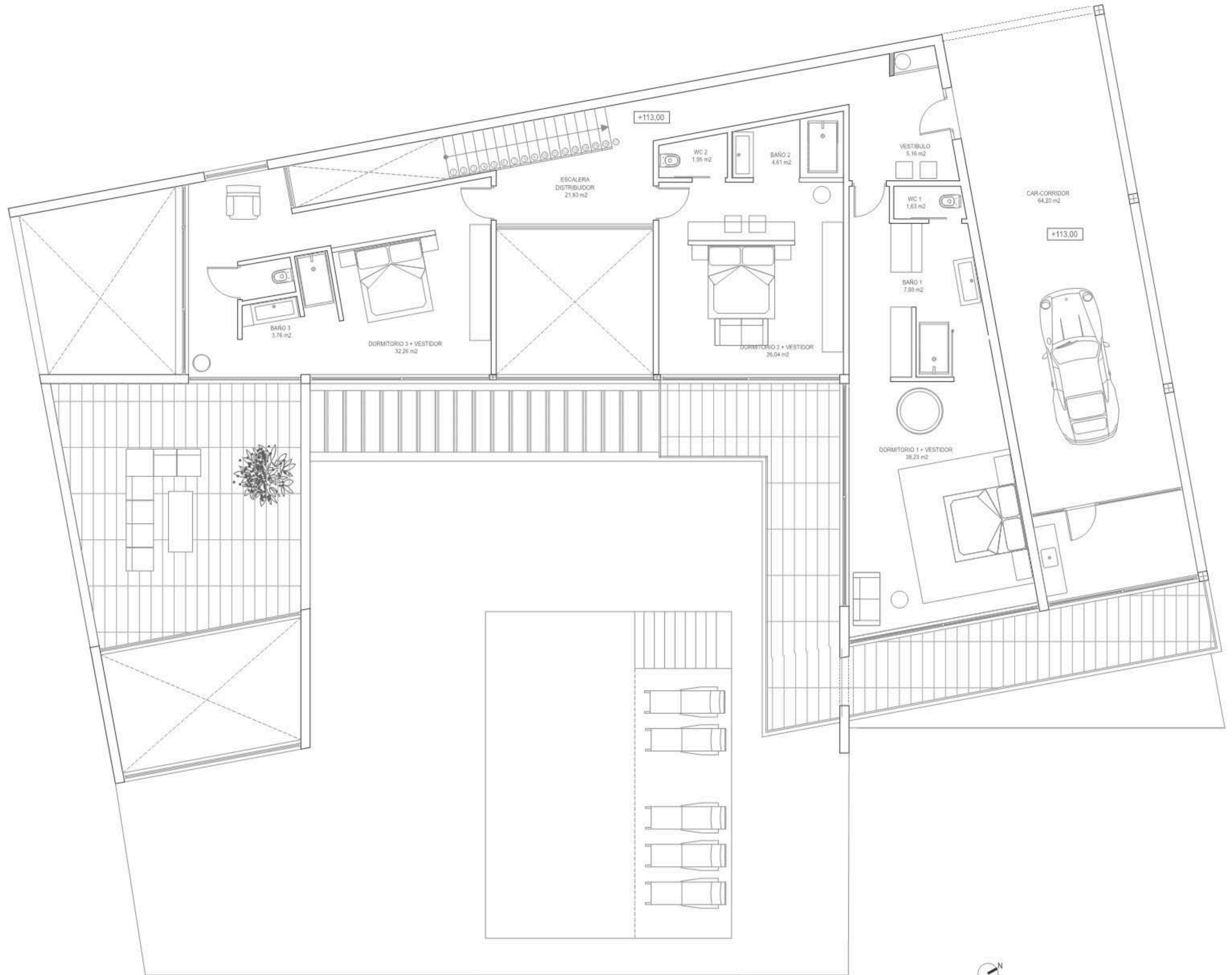
PLANTA ALTA
